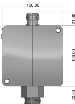
Vista frontale
